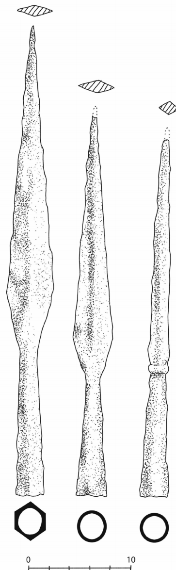
Groty włóczni z Poddębic. Pierwszy od lewej z heksagonalną tuleją – typową dla Skandynawii, pierwszy od prawej – typowy grot koczowniczy „przeciwpancerny” o kwadratowym przekroju. Rys. D. Wierzbowski
